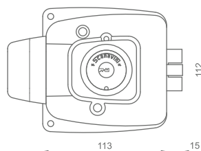
Dimensiones (mm)
